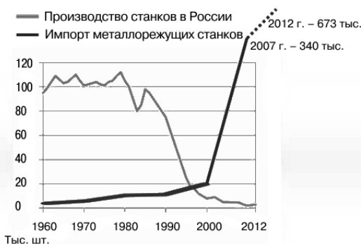
Рис. 4. Производство и импорт станков в России в 1960–2012 гг., тыс. ед.
